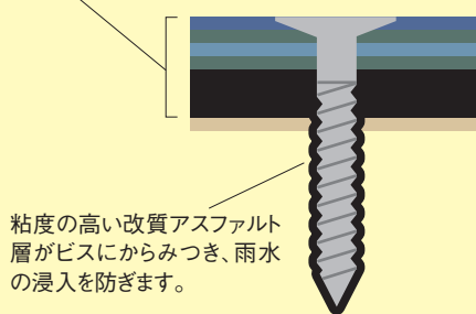
屋根下のルーフィン
