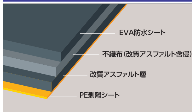
構成図
