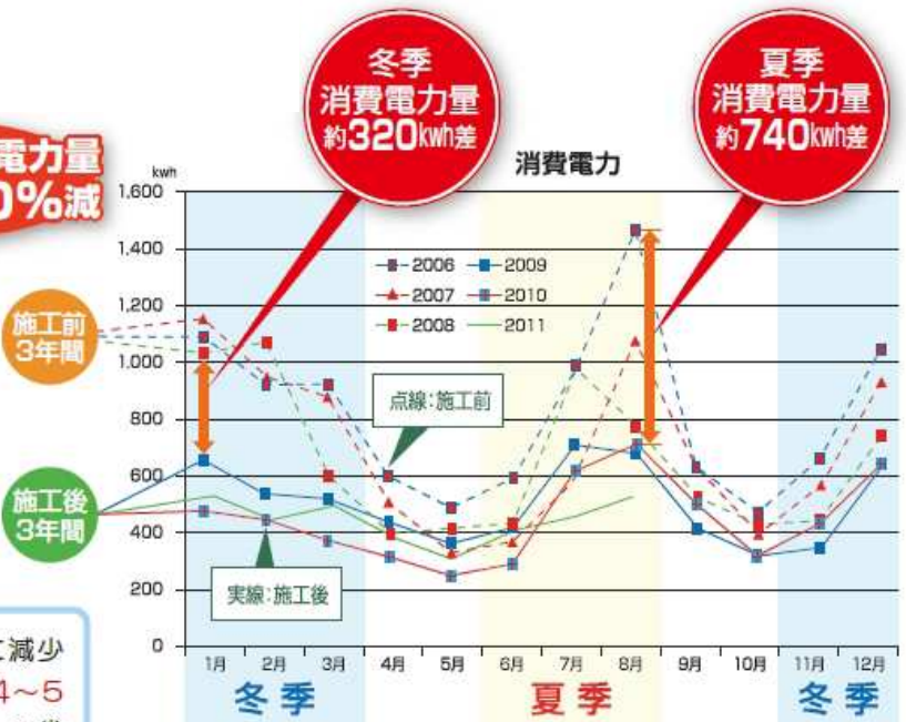
施工前後(2006年1月から2011年9月迄)の消費電力変化
