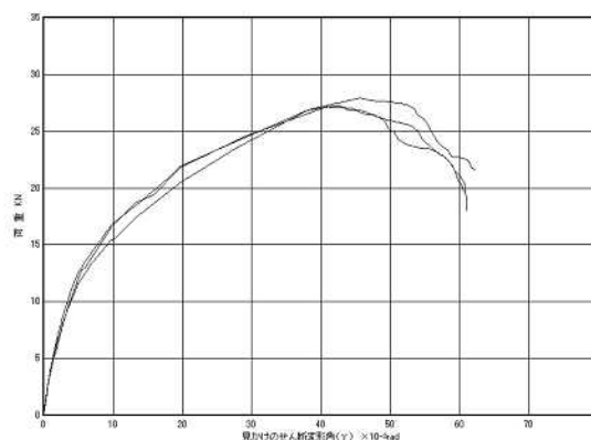
モイス大壁上部開口400mm仕様 包絡線グラフ
