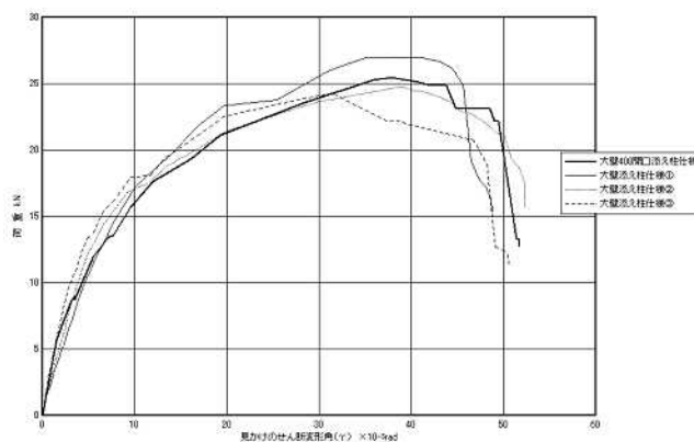
モイス大壁上部開口400mm仕様 包絡線グラフ
