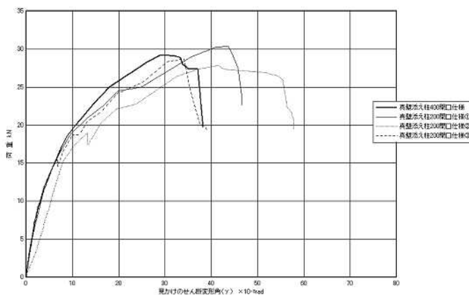
モイス真壁添え柱開口400mm仕様 包絡線グラフ
