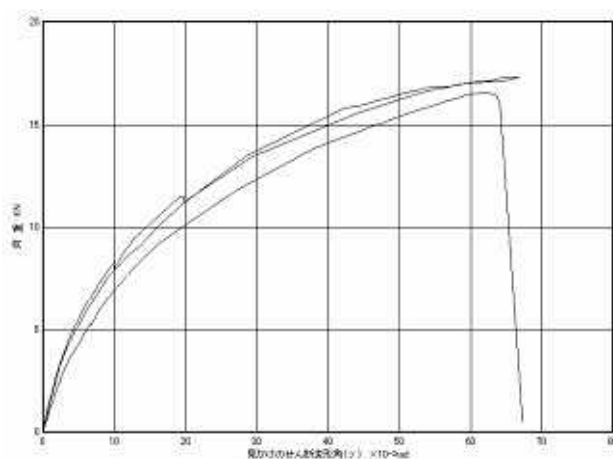
かべつよし大壁600mmスパン仕様 包絡線グラフ
